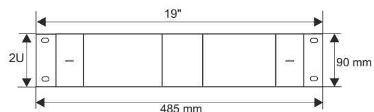
Widok z tyłu szafy RACK serii RS/ZRS
