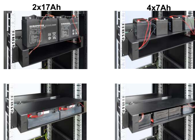
Widok z tyłu szafy RACK serii RS/ZRS
